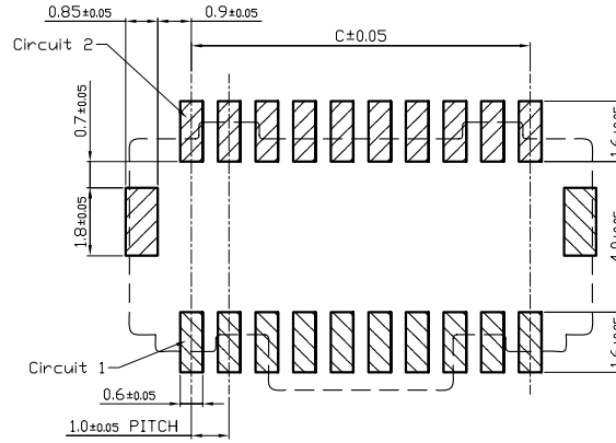
SHD-2XnAB-DK PCB寸法 PCB Layout
