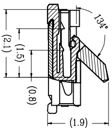
SECTION A-A SCALE 2:1
