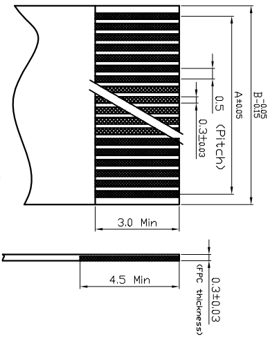
适用FPC寸法 APPLICABLE FPC
