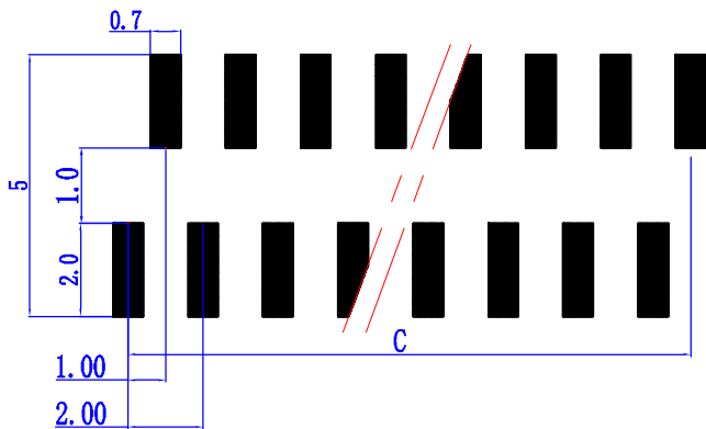
1.0-B2-nP 印制线路板 P. C. B Layout
