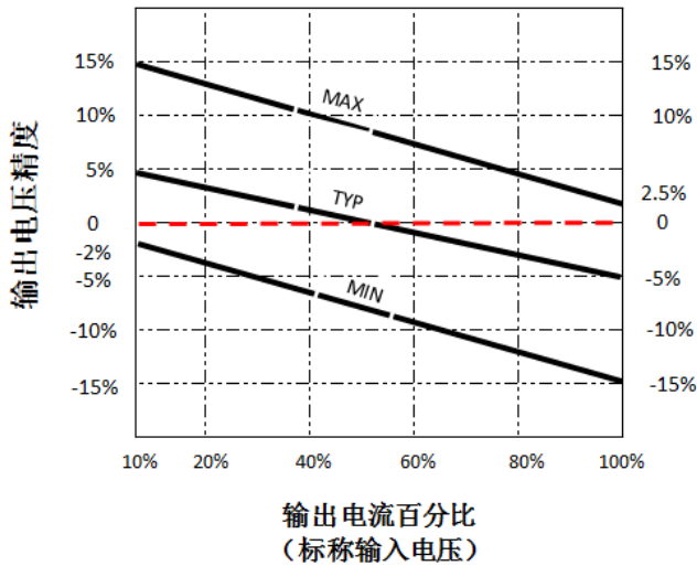
3.3V 5V输出 误差包络曲线图
