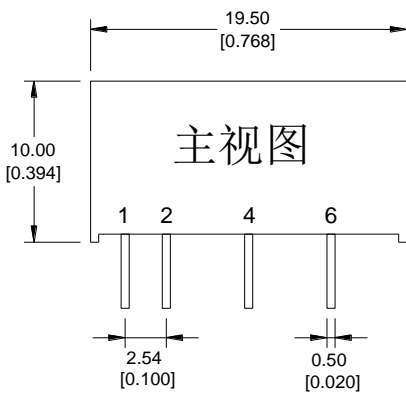
封装尺寸图
