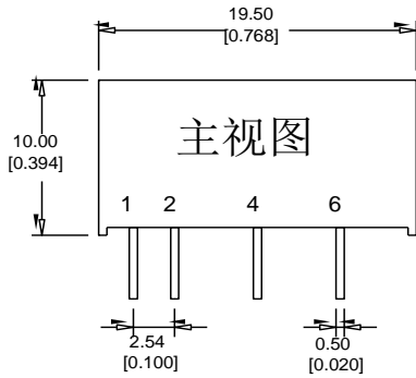
封装尺寸图
