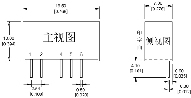
封装尺寸图
