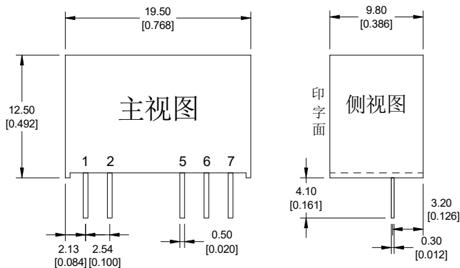
封装尺寸图
