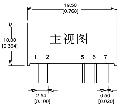
封装尺寸图
